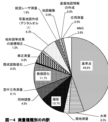
図-4 測量種類別の内訳
